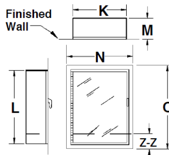
TRIMLESS
